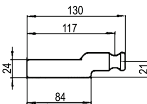
0712 159.000 Čep přímý 24x130mm H10 G Hmotnost: 0,41 kg
