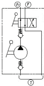
Hydraulické schéma
