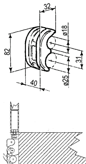
0712 407.000 Páka 40 x 82 Hmotnost : 0,2 kg
