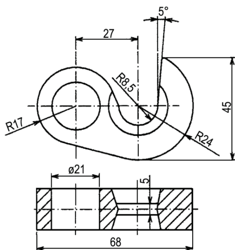
0712 229.000 Háč d=17mm Hmotnosť : 0,182 kg / ks Materiál Fe 360
